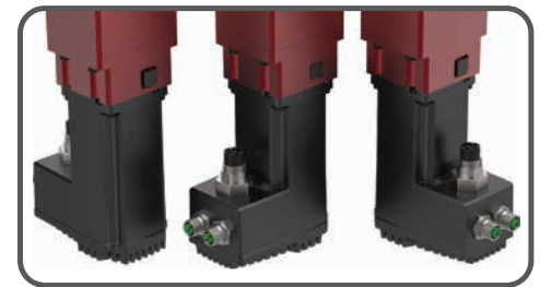
Les positions de connexion du moteur peuvent être orientées par incréments de 90°
